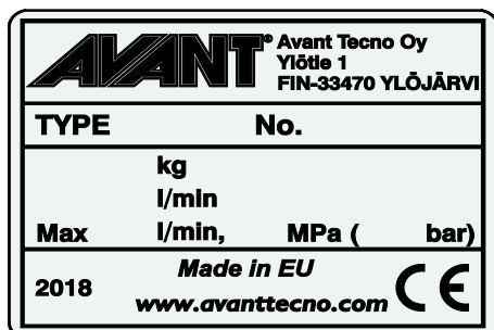
Arbetsredskapets typskylt
